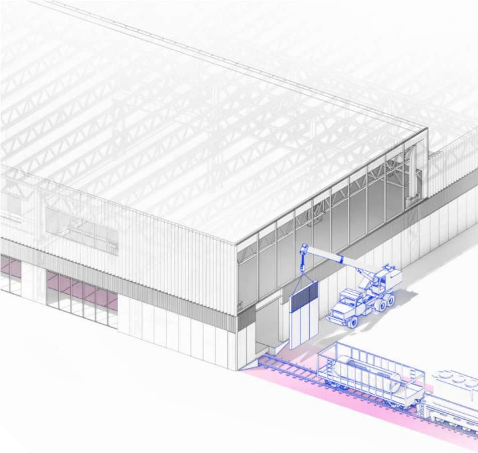
1. СНИМАЕМ ПАНЕЛИ ФАСАДА
